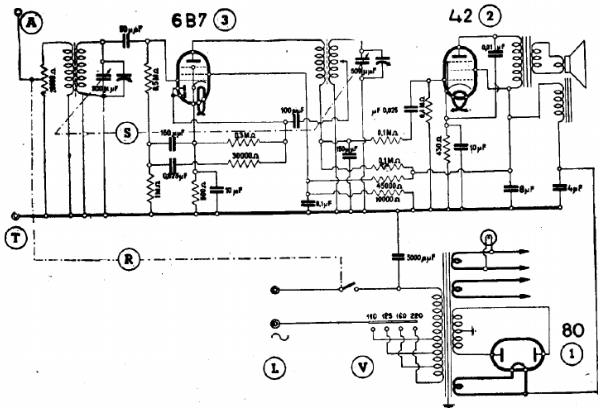
COMPAGNIA GENERALE DI ELETTRICITA' - MOD. « RADIOBALILLA »
